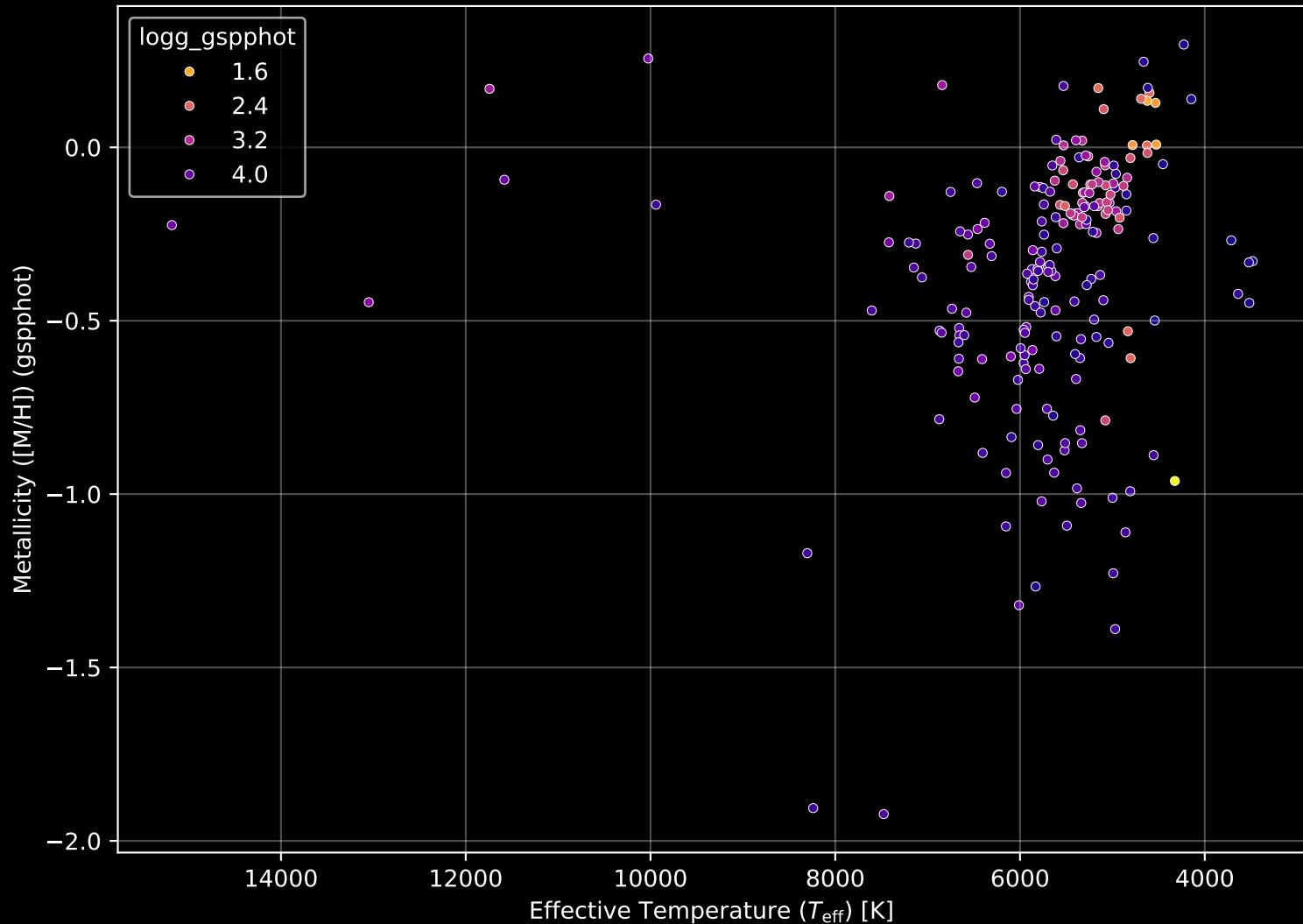
APOGEE DR17 Field: [K2_C13_180-12_btx] Stellar Population Parameters (n= 208)
